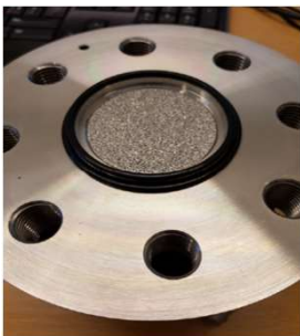
H 2 -Filter im ringförmigen Filterhalter (links) und Positioniermöglichkeit des Filterhalters im Probenahmegerät (rechts)
