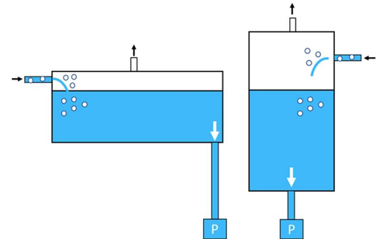
Verschiedene Bauarten von Separatoren führen zu unterschiedlicher Qualität der Gas-Flüssig-Trennung
